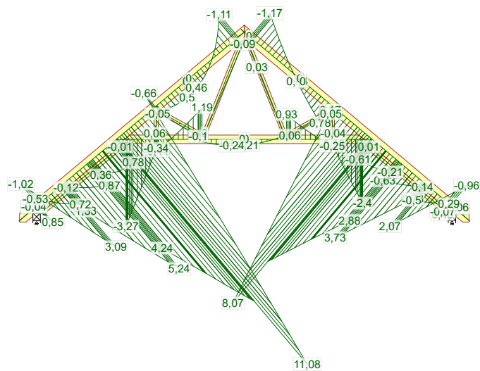
674:3 - 1,15*G+0,75*Śnieg lewy, 0 prawy+1,50*Wiatr lewy (parcie, permutacja 3)+1,05*OZ4
