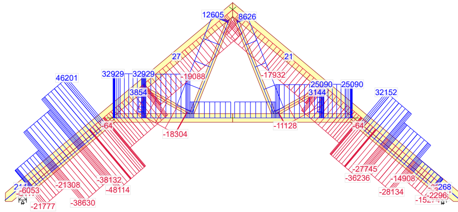
674:3 - 1,15*G+0,75*Śnieg lewy, 0 prawy+1,50*Wiatr lewy (parcie, permutacja 3)+1,05*OZ4
