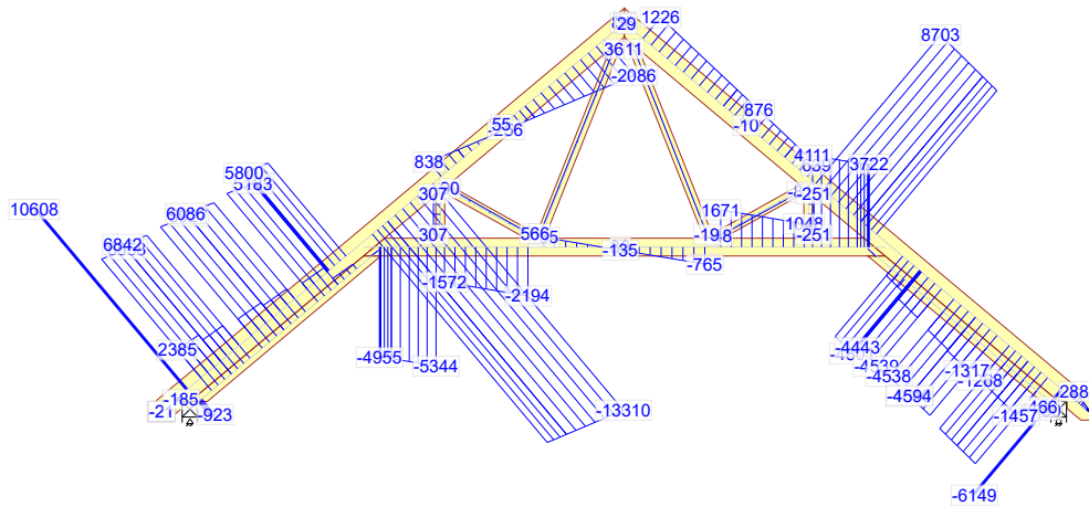
674:3 - 1,15*G+0,75*Śnieg lewy, 0 prawy+1,50*Wiatr lewy (parcie, permutacja 3)+1,05*OZ4
