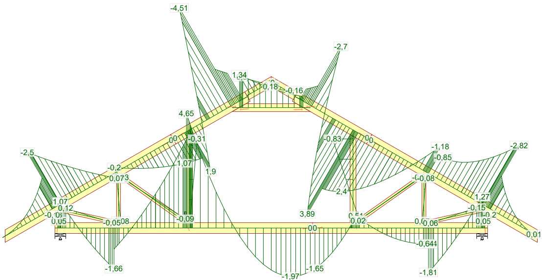
674:23 - 1,15*G+0,75*Śnieg prawy, 0 lewy+1,50*Wiatr prawy (parcie, permutacja 3)+1,05*(OZ2+OZ3)
