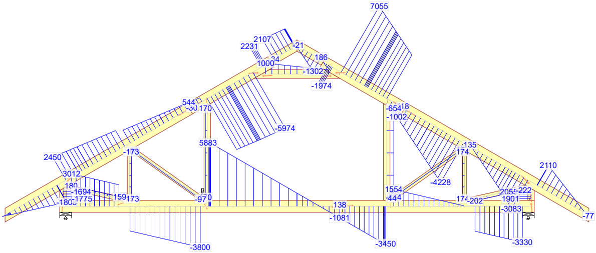
674:23 - 1,15*G+0,75*Śnieg prawy, 0 lewy+1,50*Wiatr prawy (parcie, permutacja 3)+1,05*(OZ2+OZ3)
