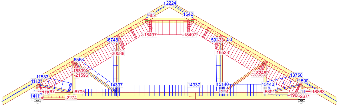
674:23 - 1,15*G+0,75*Śnieg prawy, 0 lewy+1,50*Wiatr prawy (parcie, permutacja 3)+1,05*(OZ2+OZ3)
