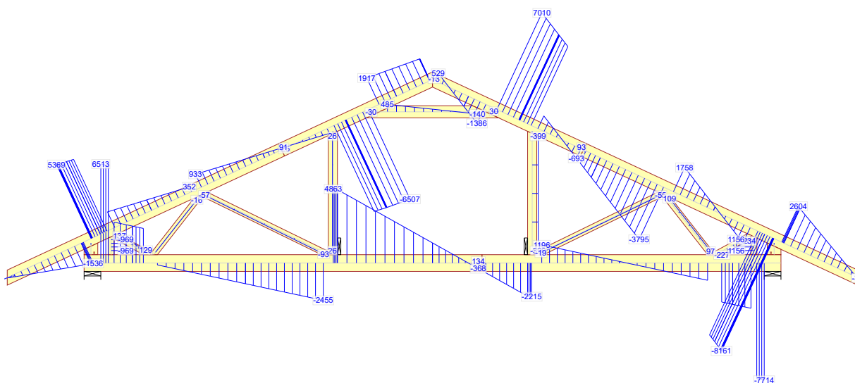
672:23 - 1,15*G+1,50*Śnieg prawy, 0 lewy+0,90*Wiatr prawy (parcie, permutacja 3)+1,05*(OZ2+OZ3)
