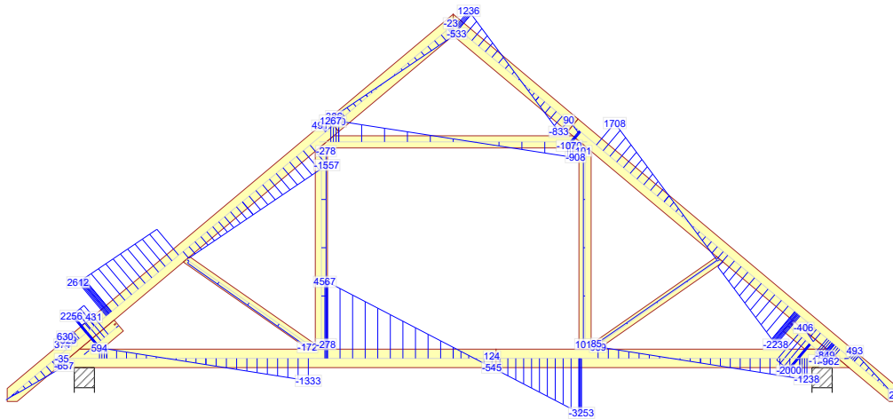
674:21 - 1,15*G+0,75*Śnieg prawy, 0 lewy+1,50*Wiatr prawy (parcie, permutacja 1)+1,05*(OZ2+OZ3+OZ4)
