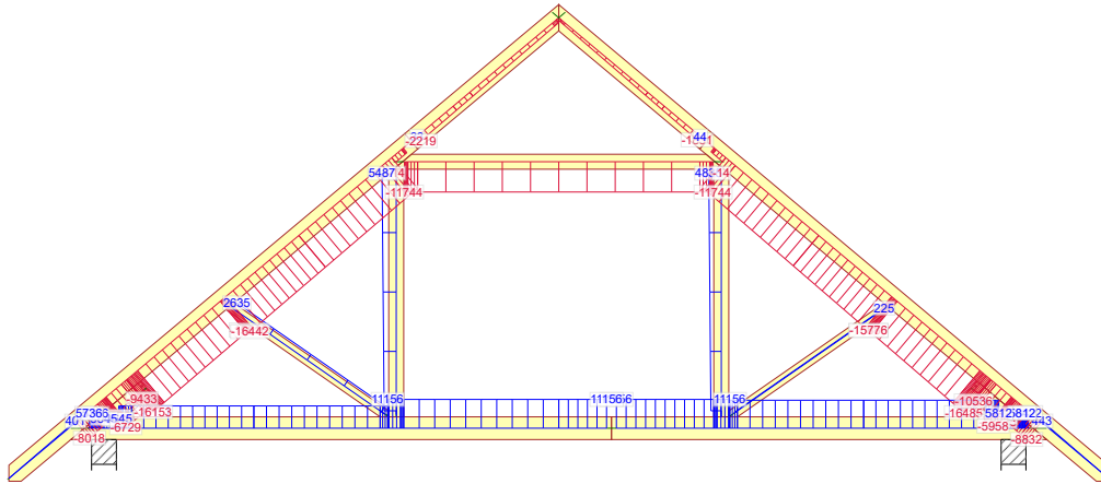
674:21 - 1,15*G+0,75*Śnieg prawy, 0 lewy+1,50*Wiatr prawy (parcie, permutacja 1)+1,05*(OZ2+OZ3+OZ4)
