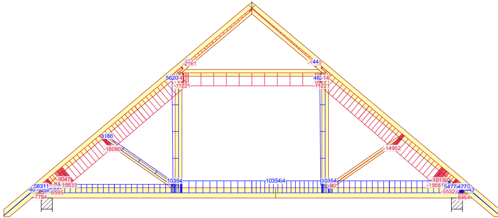
674:23 - 1,15*G+0,75*Śnieg prawy, 0 lewy+1,50*Wiatr prawy (parcie, permutacja 3)+1,05*(OZ2+OZ3+OZ4)
