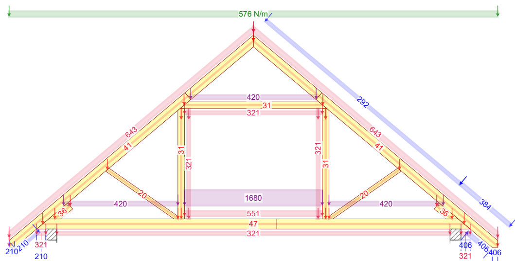
673:5 - 1,15*G+1,50*Śnieg równomiernie+0,90*Wiatr prawy (parcie, permutacja 1)+1,05*(OZ2+OZ3+OZ4)
