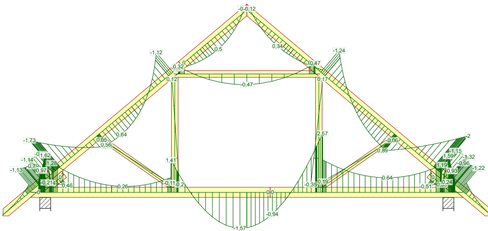
673:1 - 1,15*G+1,50*Śnieg równomiernie+0,90*Wiatr lewy (parcie, permutacja 1)+1,05*(OZ2+OZ3+OZ4)
