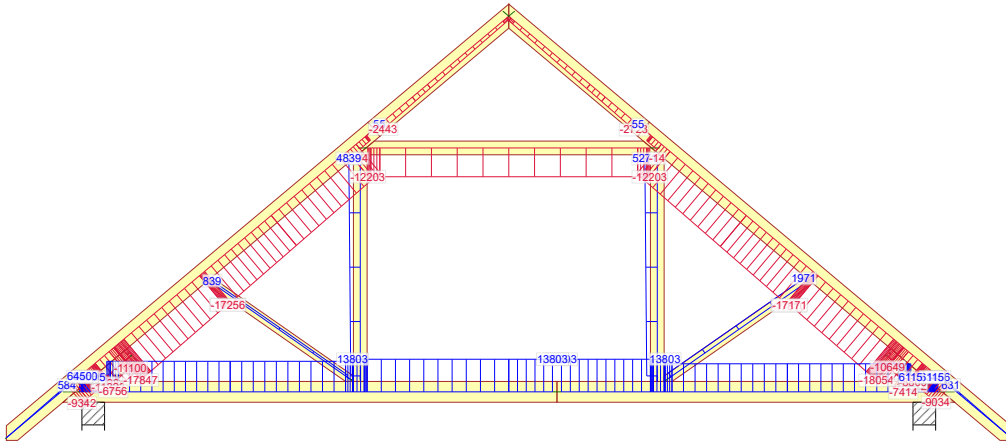
673:1 - 1,15*G+1,50*Śnieg równomiernie+0,90*Wiatr lewy (parcie, permutacja 1)+1,05*(OZ2+OZ3+OZ4)
