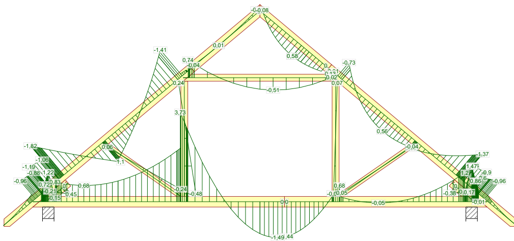
674:23 - 1,15*G+0,75*Śnieg prawy, 0 lewy+1,50*Wiatr prawy (parcie, permutacja 3)+1,05*(OZ2+OZ3+OZ4)
