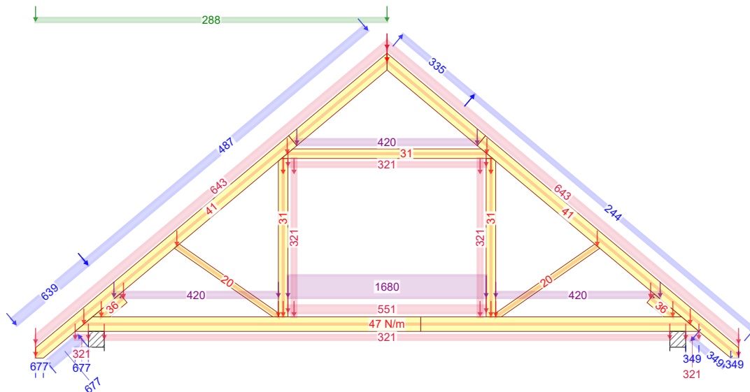
674:3 - 1,15*G+0,75*Śnieg lewy, 0 prawy+1,50*Wiatr lewy (parcie, permutacja 3)+1,05*(OZ2+OZ3+OZ4)
