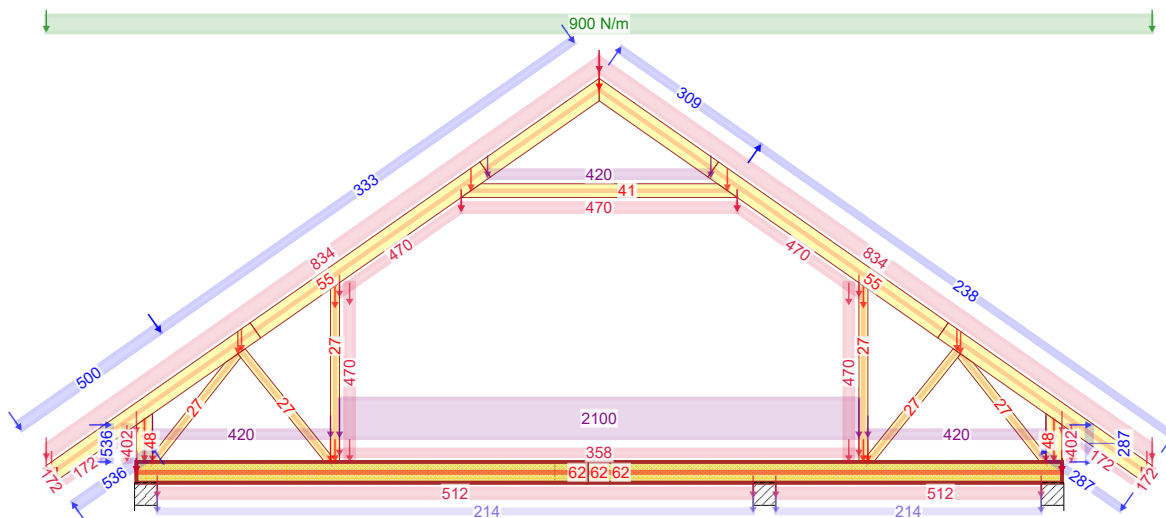
673:11 - 1,15*G+1,50*Śnieg równomiernie+0,90*Wiatr lewy (ssanie, permutacja 3)+1,05*(OZ2+OZ3+OZ4)
