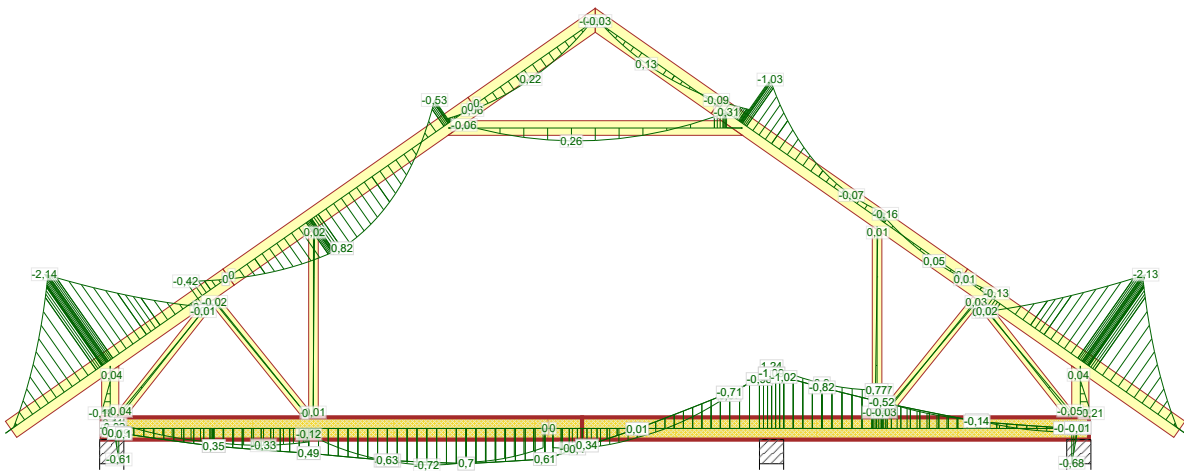
23 - 1,15*Stale + 1,50*Człowiek na wsporniku
