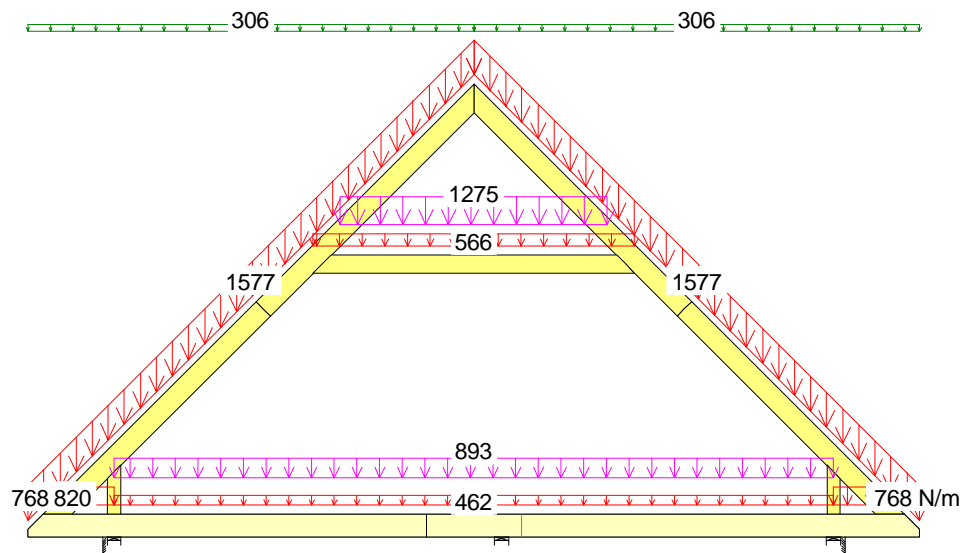
6 Śr 1.15*Stale + 0.75*Śnieg + 1.5*OZ2 + 1.05*(OZ1 + OZ3)
