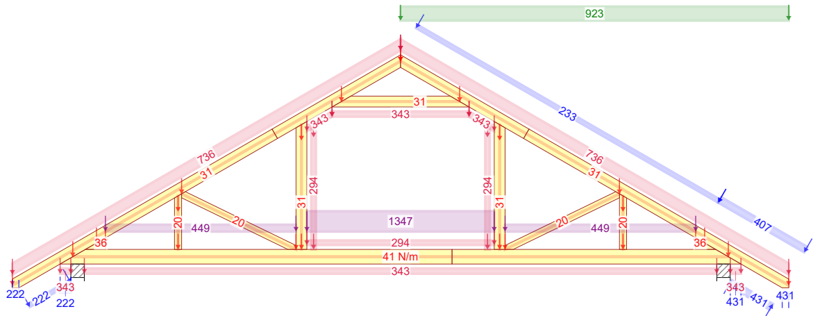
672:21 - 1,15*G+1,50*Śnieg prawy, 0 lewy+0,90*Wiatr prawy (parcie, permutacja 1)+1,05*(OZ2+OZ3)
