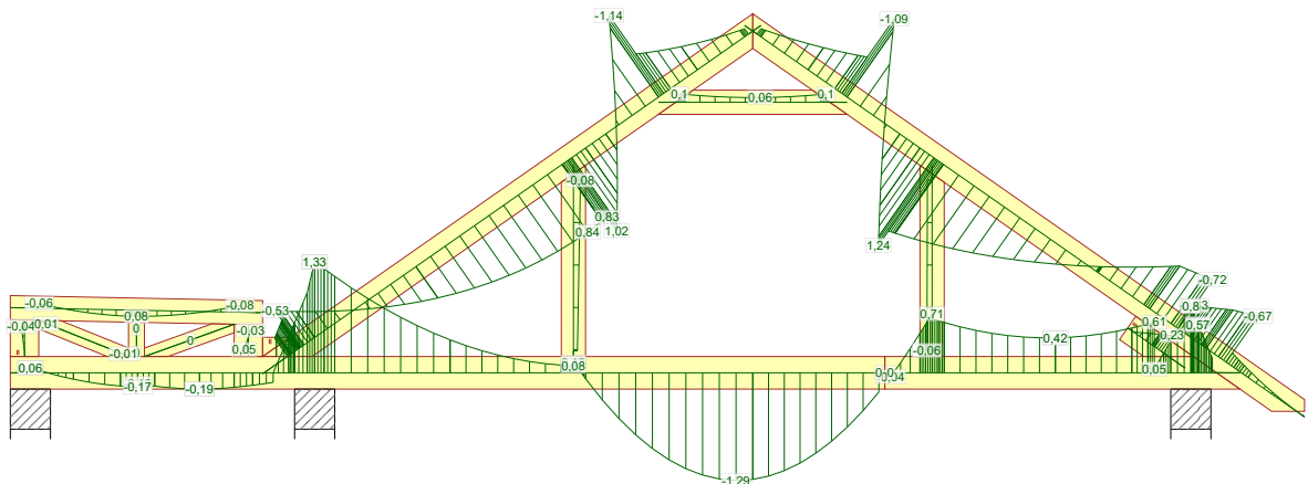
514:1 - 1,15*Stale + 0,75*Śnieg lewy ( \mu_1 lewo, 0\mu_1 prawo) + 1,05*OZ2 + 1,50*OZ3
