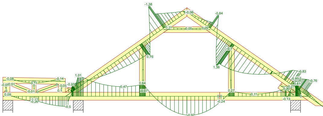
672:23 - 1,15*G+1,50*Śnieg prawy, 0 lewy+0,90*Wiatr prawy (parcie, permutacja 3)+1,05*(OZ2+OZ3)
