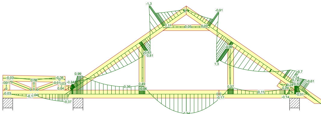
674:7 - 1,15*G+0,75*Śnieg lewy, 0 prawy+1,50*Wiatr prawy (parcie, permutacja 3)+1,05*(OZ2+OZ3)
