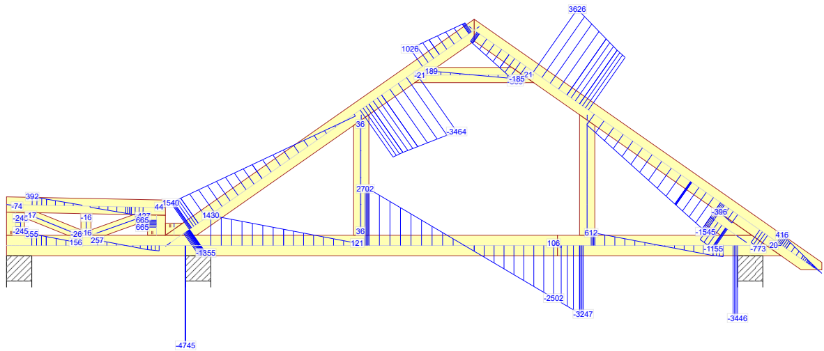
514:1 - 1,15*Stale + 0,75*Śnieg lewy ( \mu_1 lewo, 0\mu_1 prawo) + 1,05*OZ2 + 1,50*OZ3
