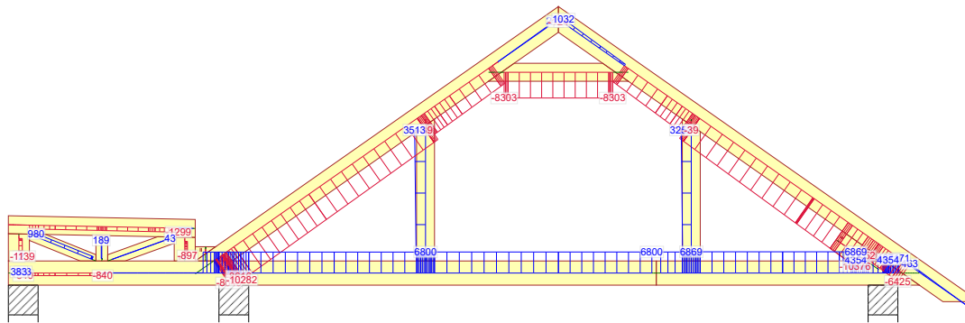
672:23 - 1,15*G+1,50*Śnieg prawy, 0 lewy+0,90*Wiatr prawy (parcie, permutacja 3)+1,05*(OZ2+OZ3)
