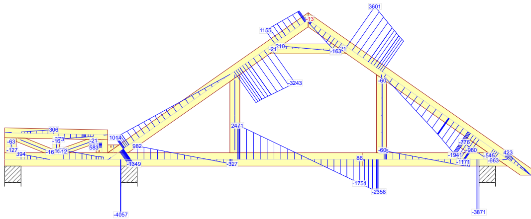
674:7 - 1,15*G+0,75*Śnieg lewy, 0 prawy+1,50*Wiatr prawy (parcie, permutacja 3)+1,05*(OZ2+OZ3)
