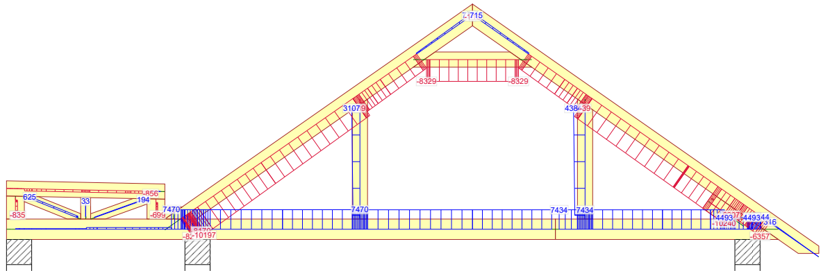
514:1 - 1,15*Stale + 0,75*Śnieg lewy ( \mu_1 lewo, 0\mu_1 prawo) + 1,05*OZ2 + 1,50*OZ3
