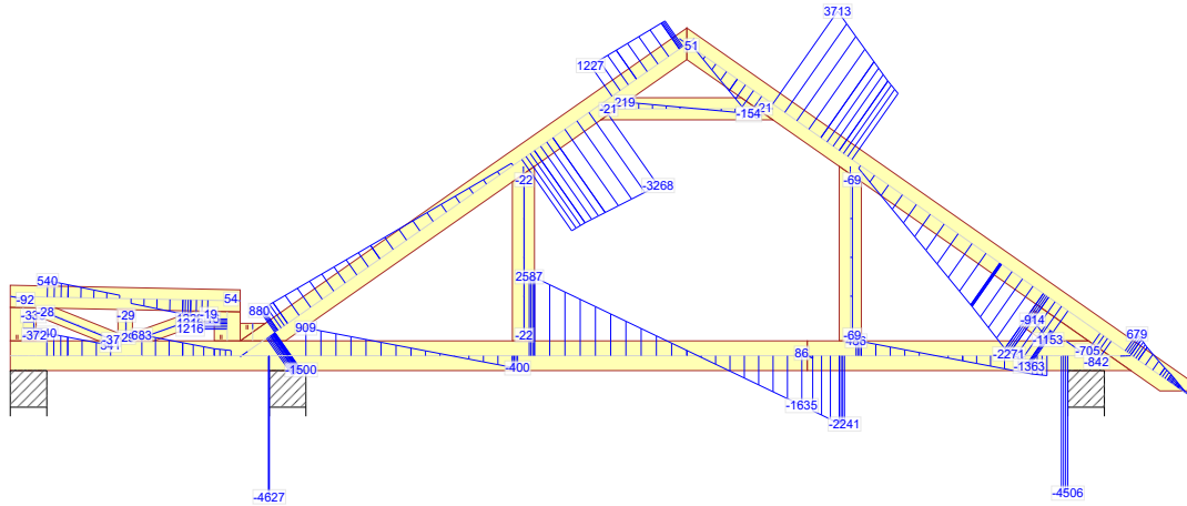
672:23 - 1,15*G+1,50*Śnieg prawy, 0 lewy+0,90*Wiatr prawy (parcie, permutacja 3)+1,05*(OZ2+OZ3)
