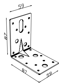
Kątownik HD 90 90 łącznik więzarów i legarów z podwaliną (190 szt.)
