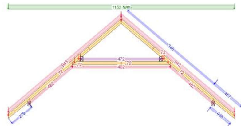
Stan Graniczny Nośności - Krótkotrwale
