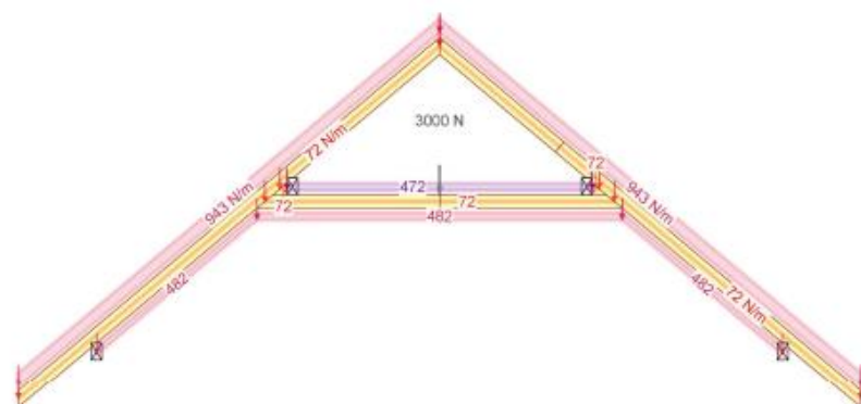
Stan Graniczny Nośności - Chwilowe
