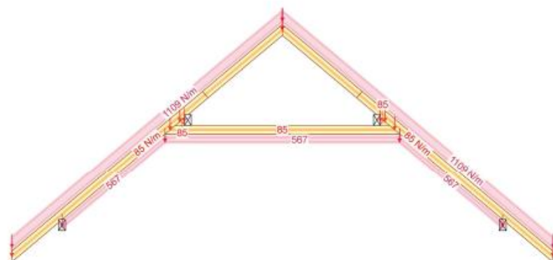
Stan Graniczny Nośności - Stałe
