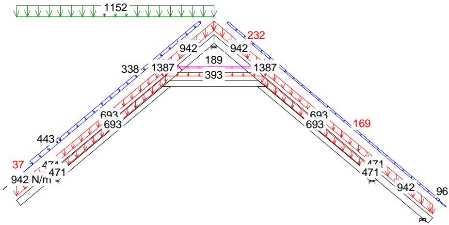
13 Kr 1.15*Stałe, 1.5*ŚniegL(0 P), 1.05*Wiatr LS, 1.05*OZ
