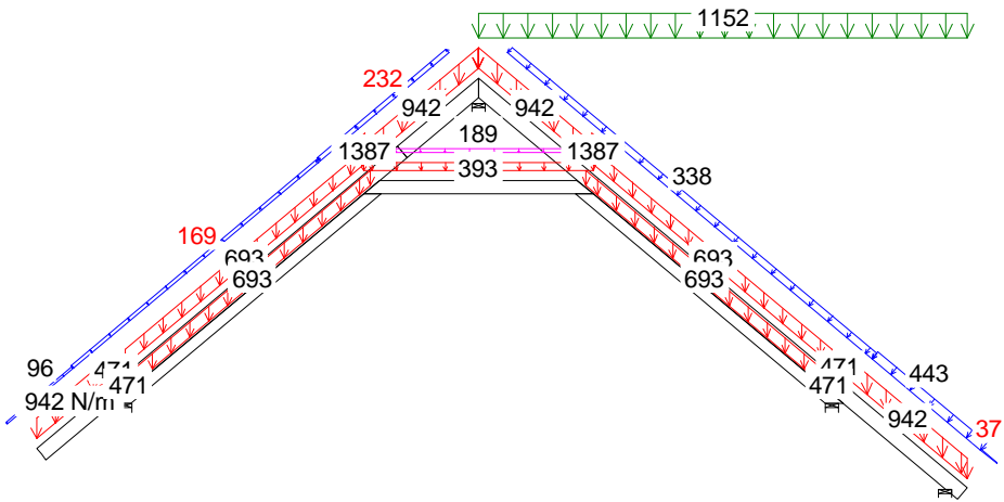
14 Kr 1.15*Stałe, 1.5*ŚniegP(0 L), 1.05*Wiatr PS, 1.05*OZ
