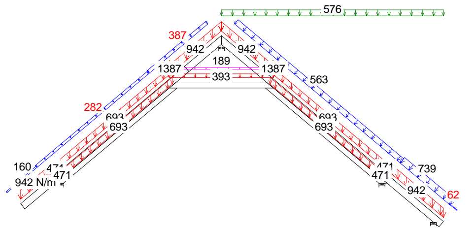
16 Kr 1.15*Stałe, 1.05*ŚniegP(0 L), 1.5*Wiatr PS, 1.05*OZ
